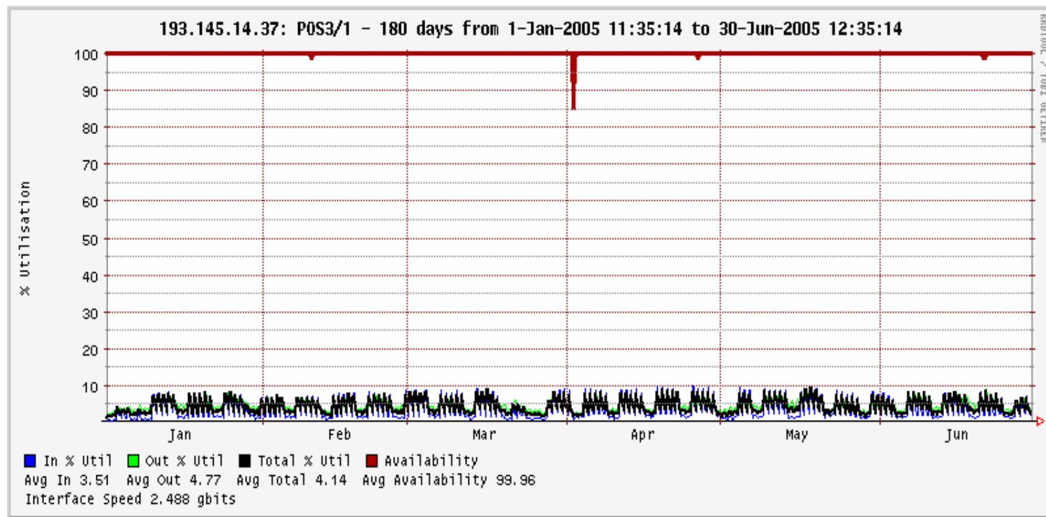
Figura 3: utilización del enlace con RedIRIS a 2.5 Gbps
