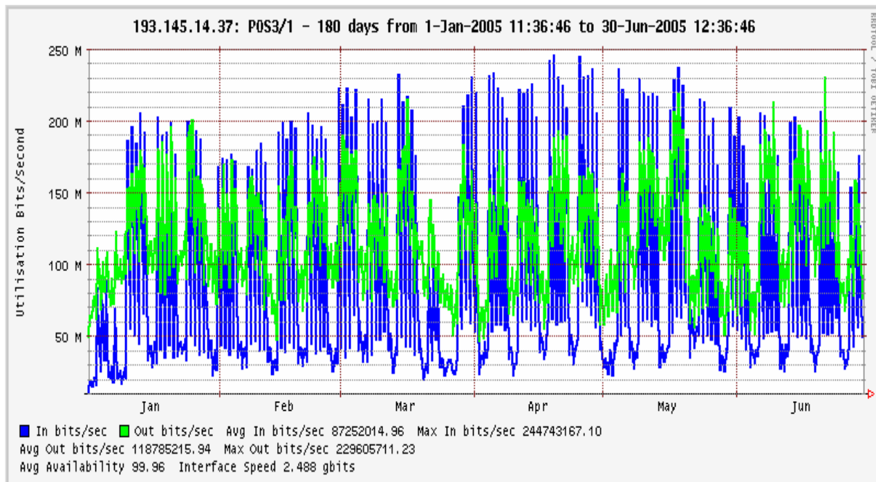
Figura 4: tráfico encaminado por el enlace con RedIRIS a 2.5 Gbps
