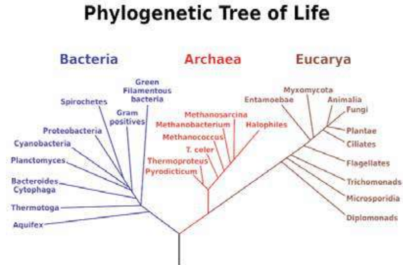
Figura 29: Árbol filogenético.
