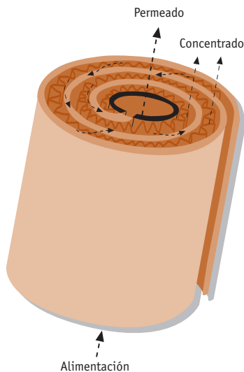
FIGURA 3.5 Membrana enrollada en espiral.
